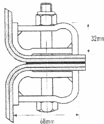
Typ2 < 800 kN/m
